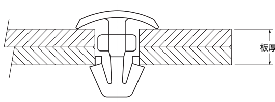
取付状態図
