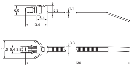
図1：プッシュマウントタイ
